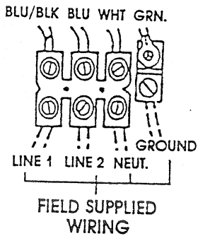
240 VOLT WIRING DIAGRAM
